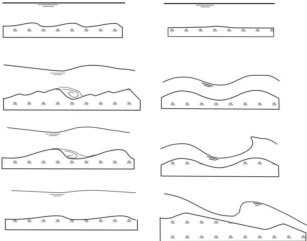
Figura 3.16: Ondas sedimentarias del tipo micro y mesoformas.
